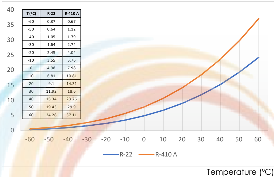
Gráfico Presión - Temperatura (°C) Pressure (bar)
